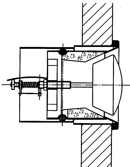
Einbau mit Mauerrahmen
