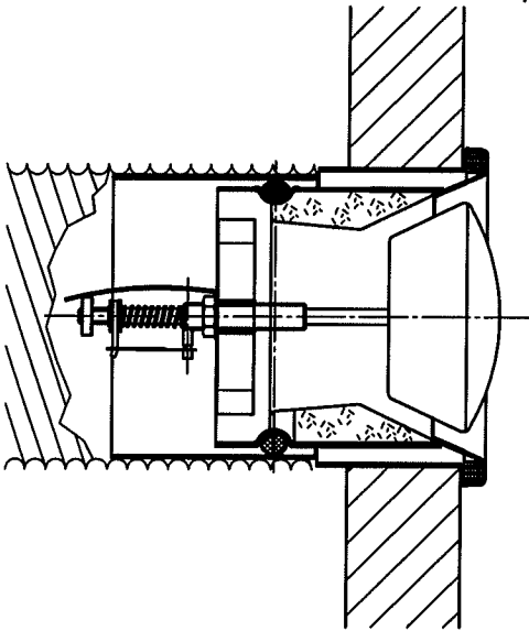
Einbau mit Mauerrahmen und angeschlossenem Flexschlauch.
