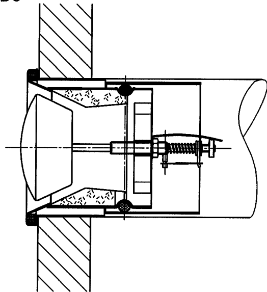
Einbau mit Mauerrahmen und angeschlossener, brennbarer Rohrleitung
