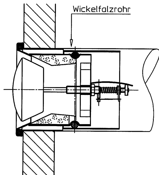
Einbau mit Mauerrahmen und Normwickelfalzrohr
