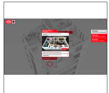
Helios_Heliosphere_2.jpg
